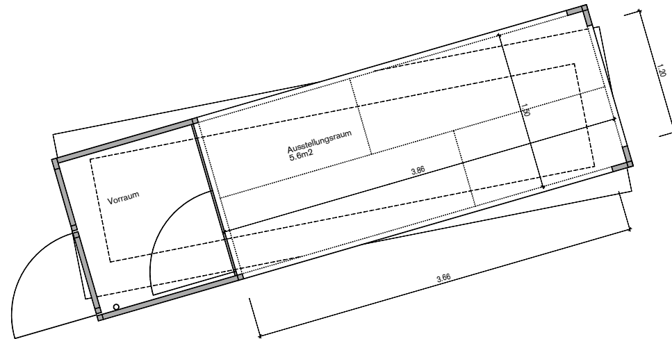
Grundriss Kunstkasten
