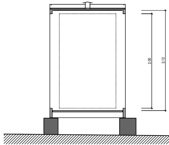
Querschnitt Kunstkasten
